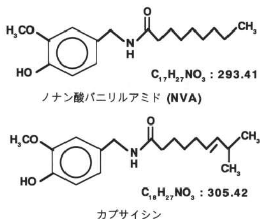
図6 NVAとカプサイシンの化学構造式
