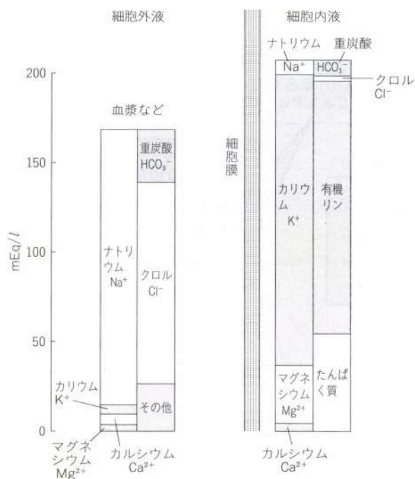
図11 イオン組成
